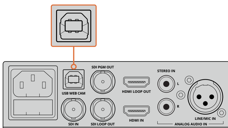
将Blackmagic Web Presenter通过后面板的USB端口连接电脑
