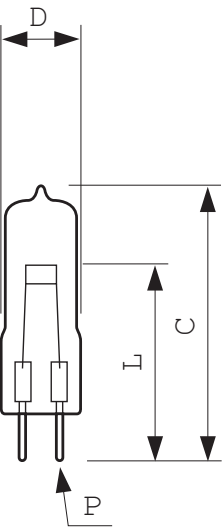
7158 150W G6.35 24V 1CT
